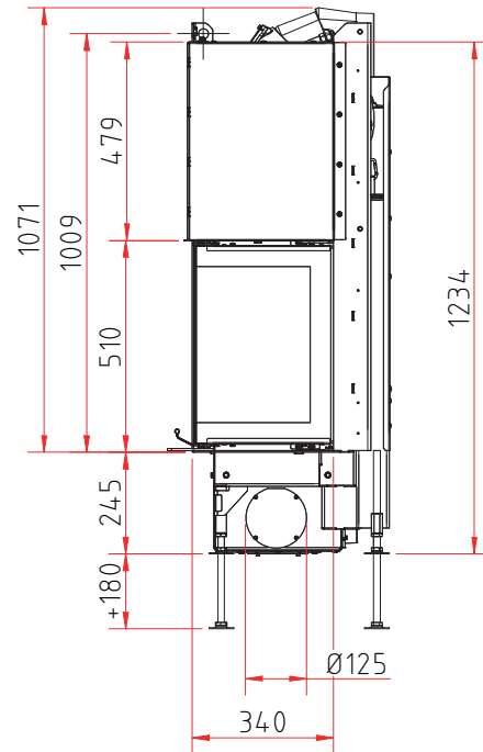
Seitenansicht M 1:20
