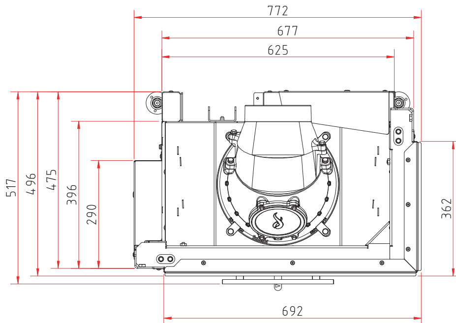
Draufsicht M 1:10
