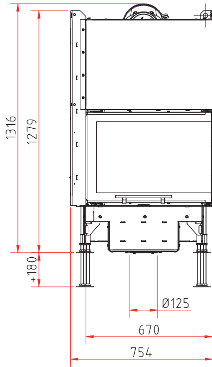
Frontansicht M 1:20
