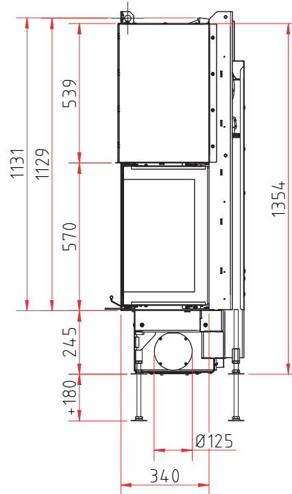
Seitenansicht M 1:20
