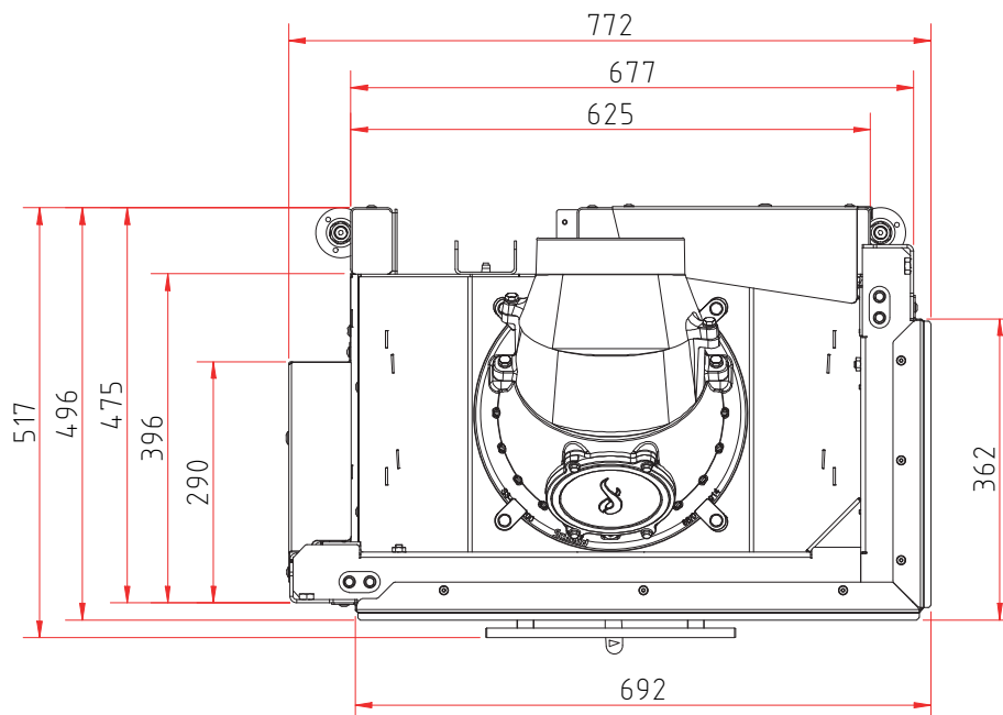
Draufsicht M 1:10
