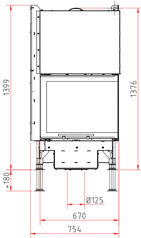
Frontansicht M 1:20
